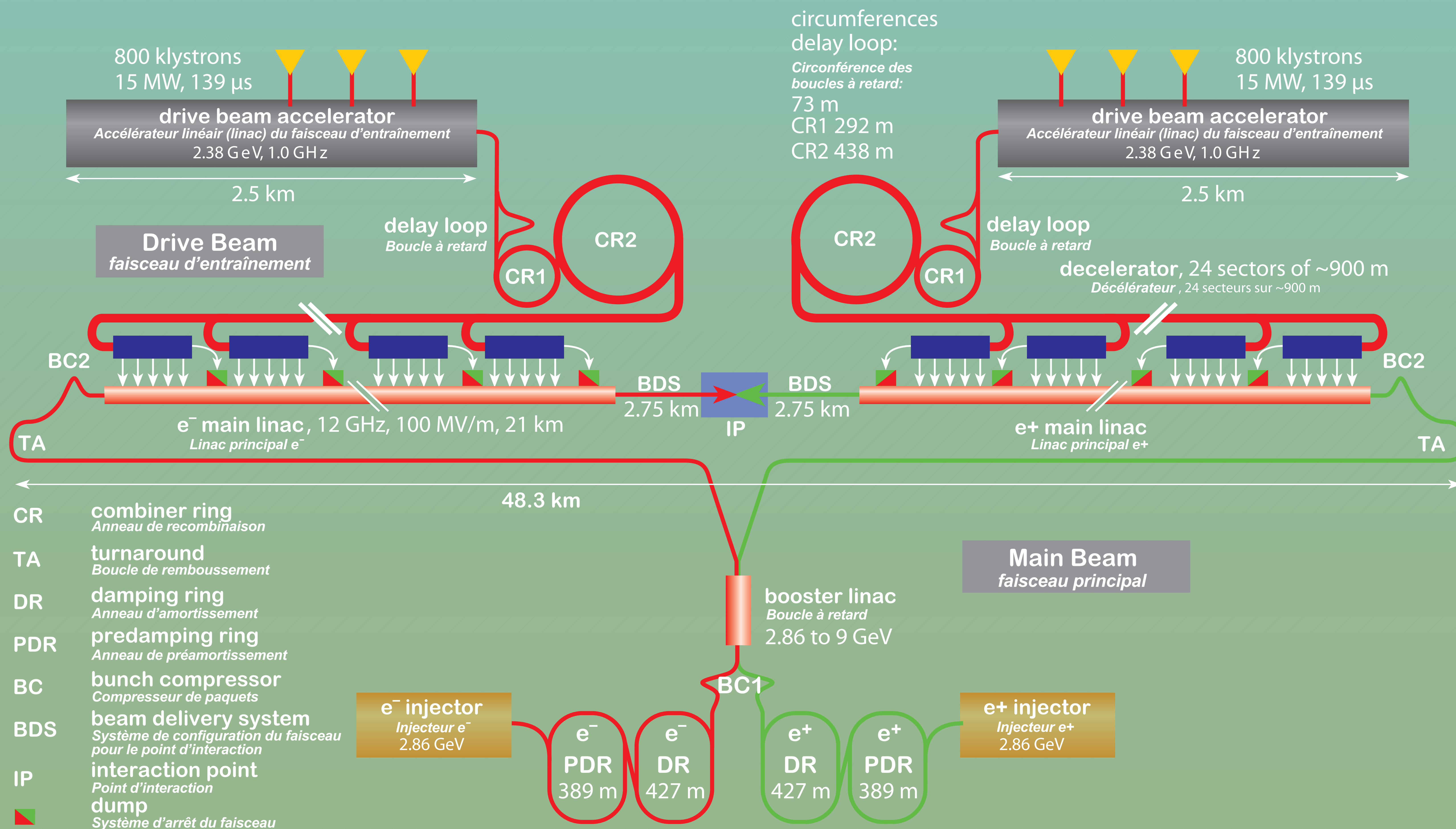
CLIC overall layout Schéma général de CLIC
